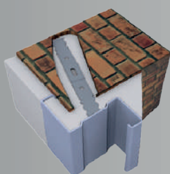
INSTALLAZIONE CON ARTIGLI INSTALLATION AVEC DES GRIFFES
