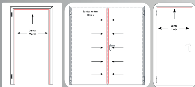
GUARNIZIONI PER FUMI JOINTS ANTI-FUMÉE
